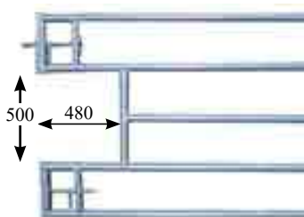
Handel grind med uttag för hängande vattenkopp. Art nr. LV5 - 125315
