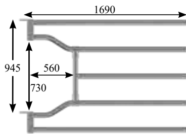
Handel med uttag för hängande vattenkopp. Art nr. LV4 - 124250 Art nr. LV5 - 125310
