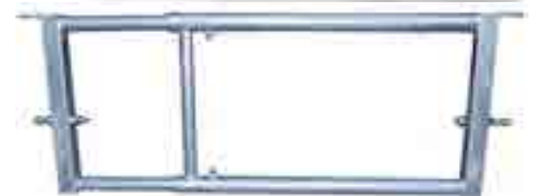
Grind LV2 med två liggande rör Ø60/49 mm. Finns i längder 1-2, 2-3, 3-4, 4-5 och 5-6 m.
